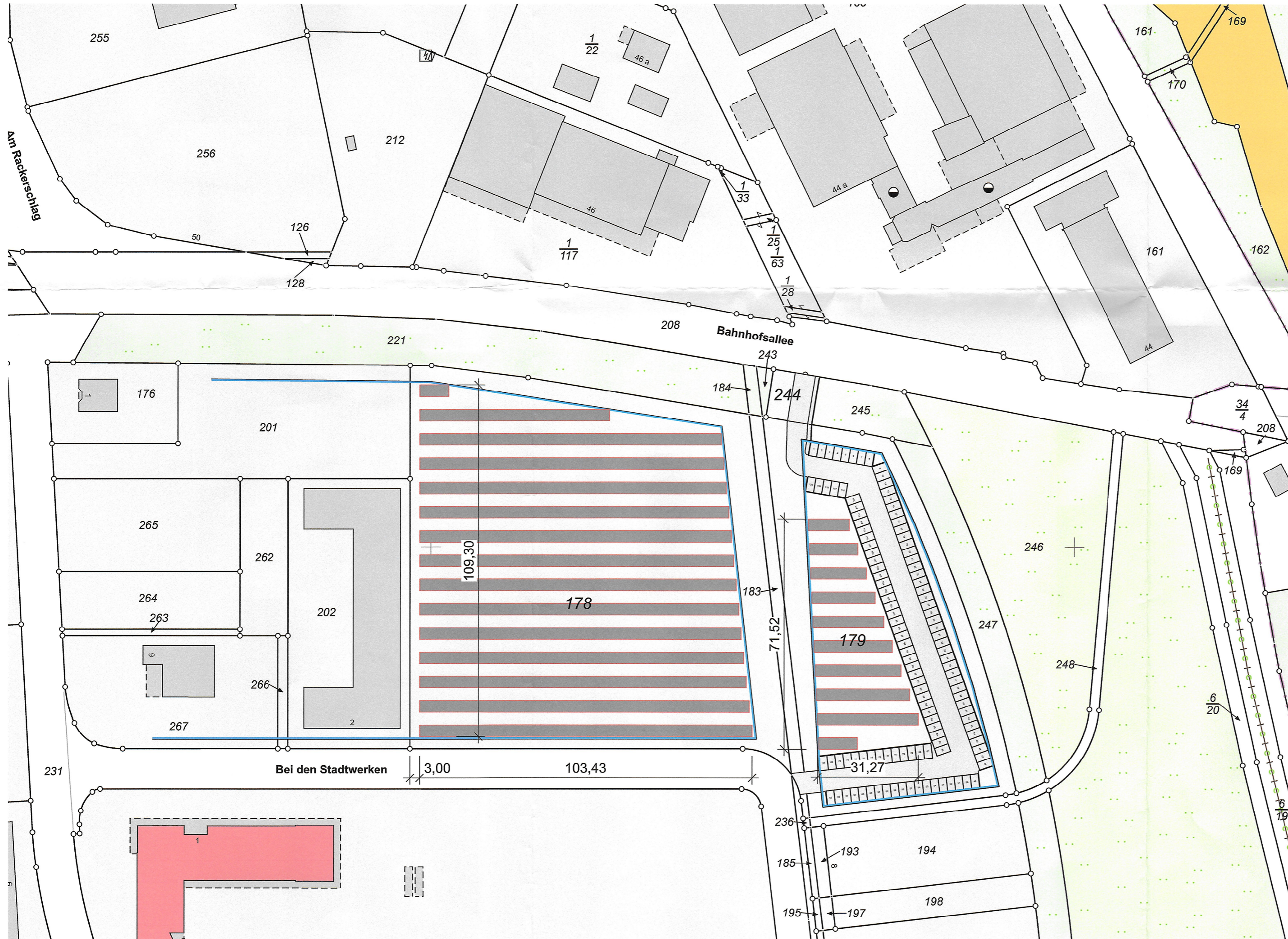
Lageplan, M 1: 1000
